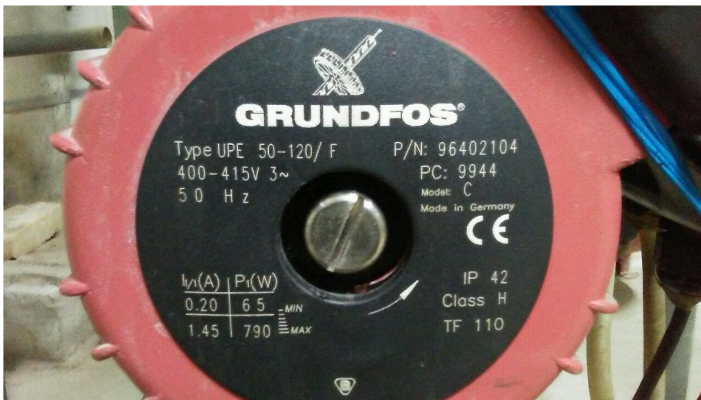
Zdjęcie 2. Tabliczka znamionowa pompy do wymiany.
